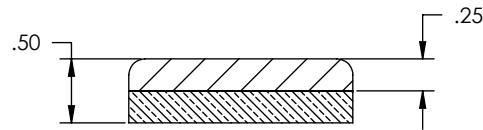
SECTION A-A SCALE 1 : 1.5
